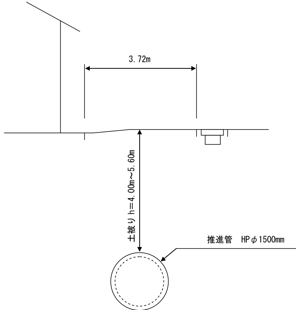
横断図
