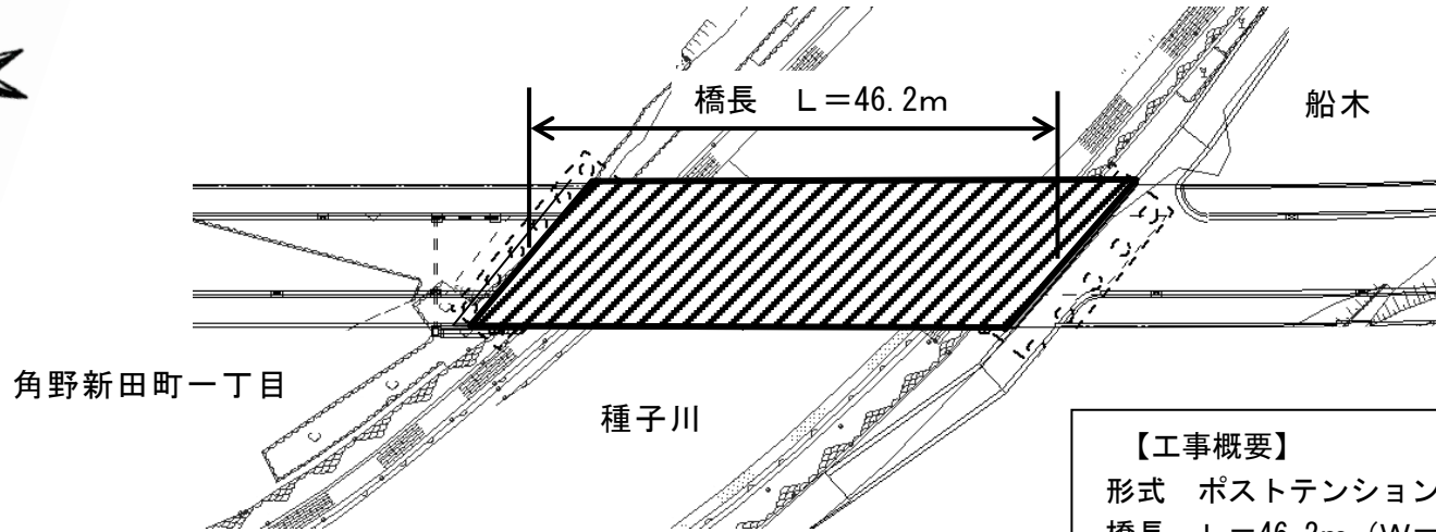
平面図
