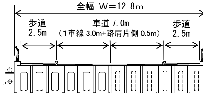
断面図
