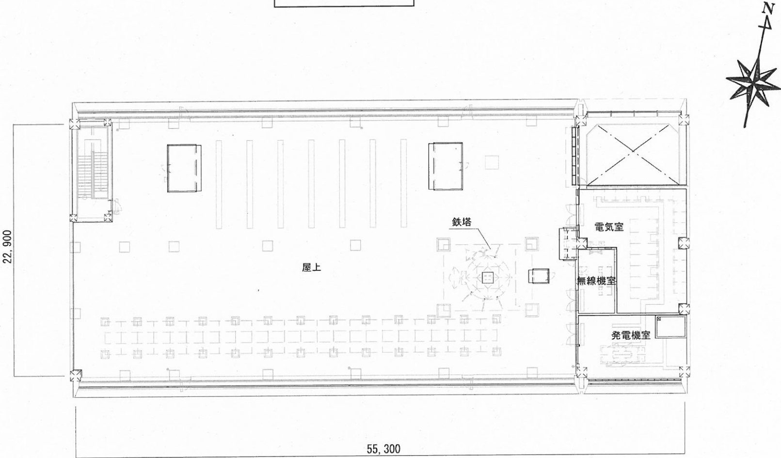
6階平面図
