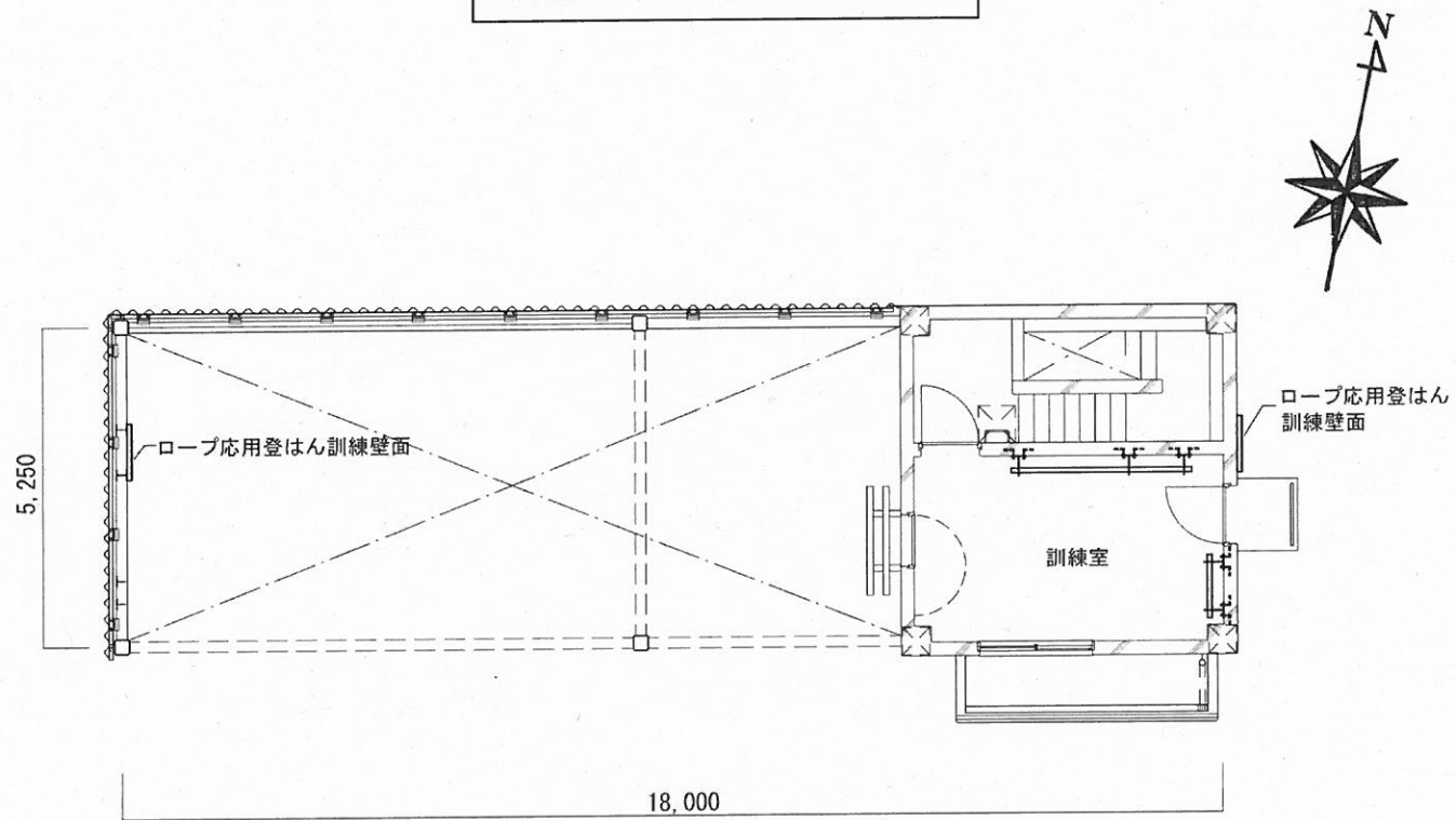
訓練棟 主塔5階平面図
