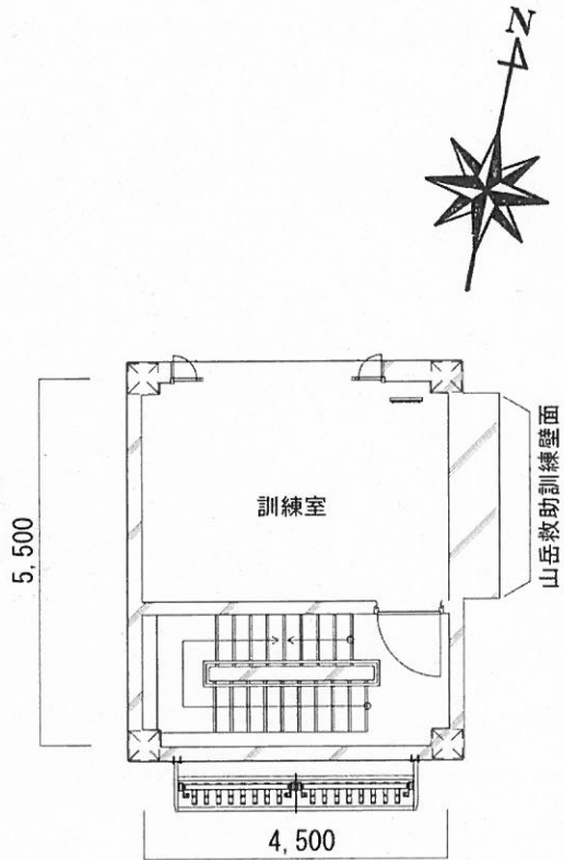
訓練棟 副塔 2階平面図
