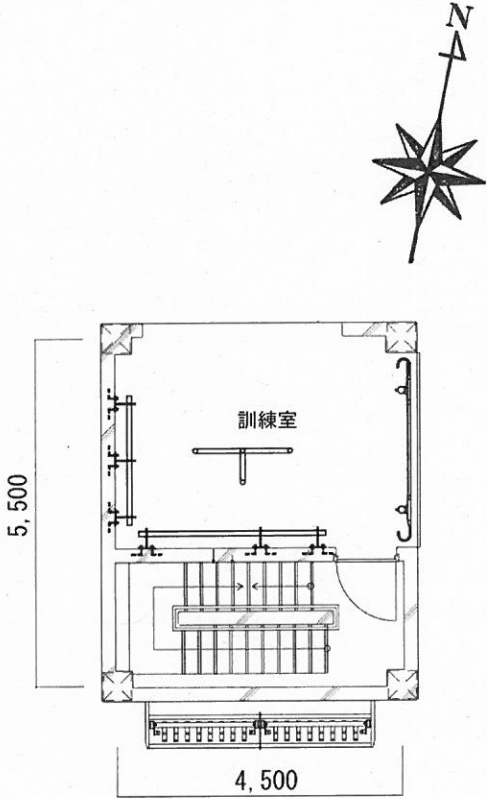
訓練棟 副塔3階平面図
