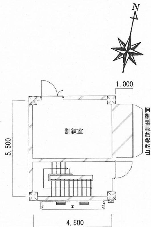
訓練棟 副塔 1階平面図
