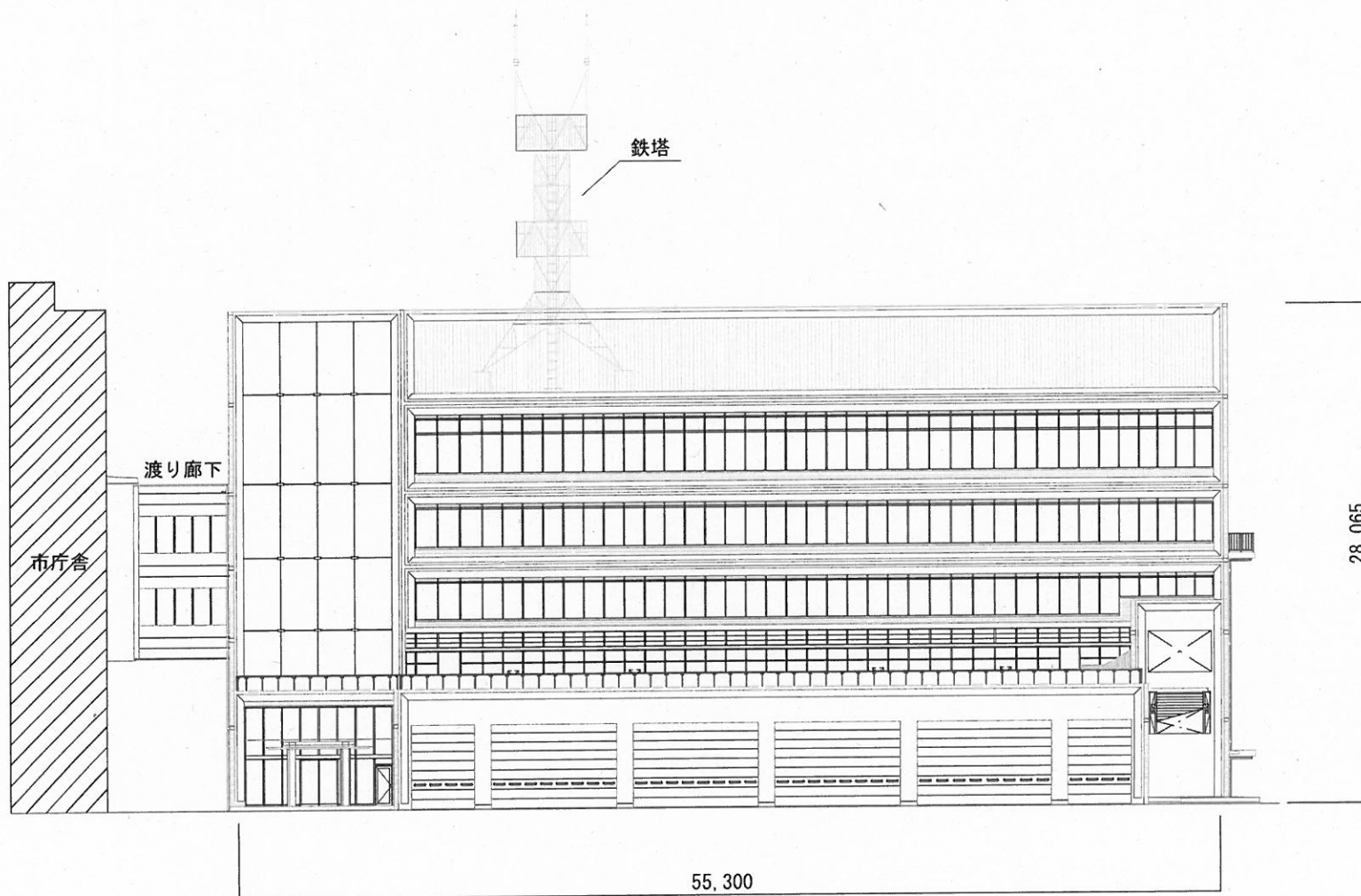
北立面図
