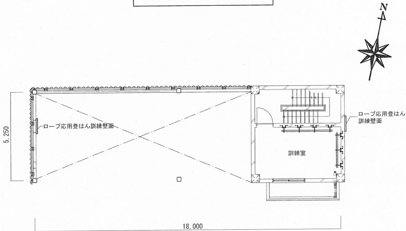
訓練棟 主塔4階平面図
